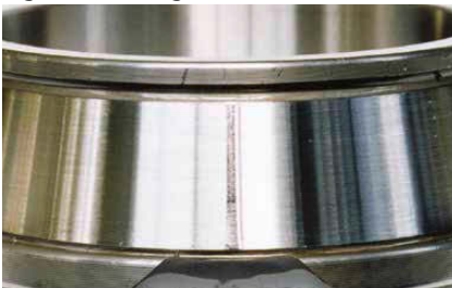
Fig. 30: Fracture
