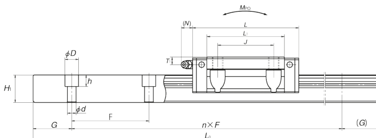
SIDE VIEW OF EM TYPE
