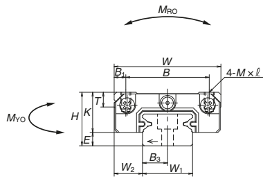
RAIL OF PU TYPE
